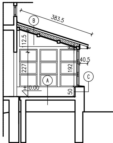
PRZEKRÓJ C - C
